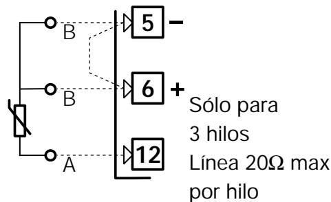
Para termoresistencia Pt100
