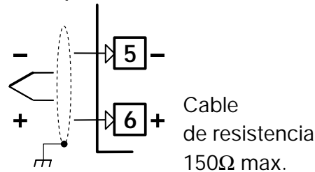
Termopar L-J-K-S-T
