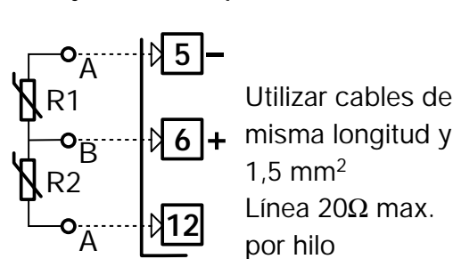
Para ejecuciones especiales ΔT (2x Pt100)
